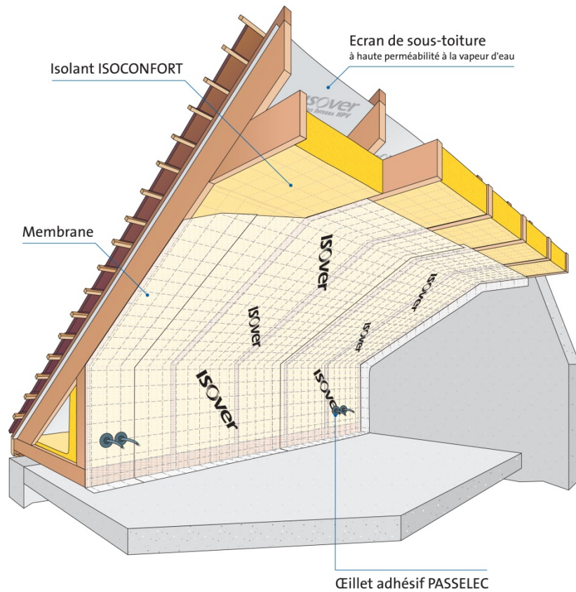
Figure 6 - Charpente en fermettes industrialisées pour comble aménagé : Passage de gaines au travers de la membrane
