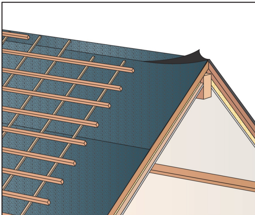
Figure 48 - Traitement du faîtage : raccordement de l'écran de sous-toiture au niveau de la ligne de faîtage à la fin du second versant
