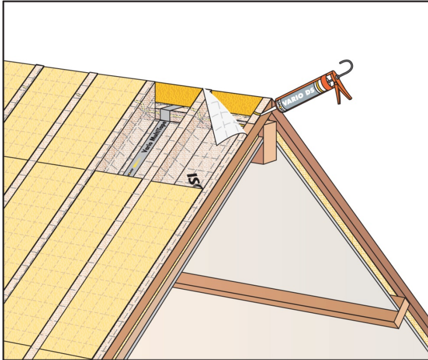
Figure 47 - Traitement du faîtage : scellement au mastic VARIO DS des deux membranes lors de la fin du traitement du second versant
