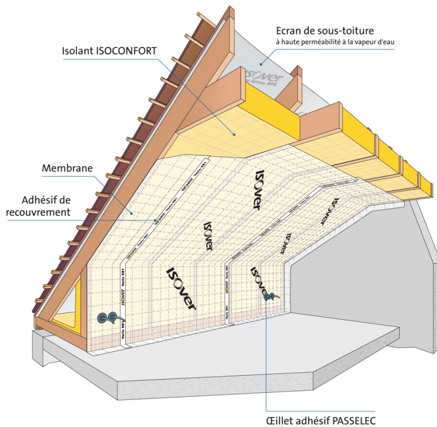
Figure 7 - Charpente en fermettes industrialisées pour comble aménagé : Jointoiment des lés de membrane
