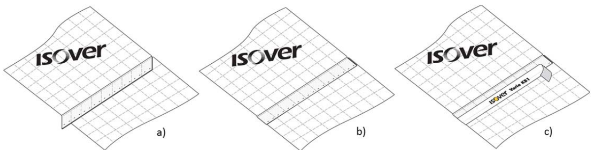
Figure 17 - Charpente en fermettes industrialisées pour comble perdu : Isolant en vrac soufflé mécaniquement - Mise en œuvre du procédé avec la suspenste Intégra2 – focus sur la jonction des lès de membrane – vue de dessous (a) agrafage, (b) pliage, (c) pose de l'adhésif
