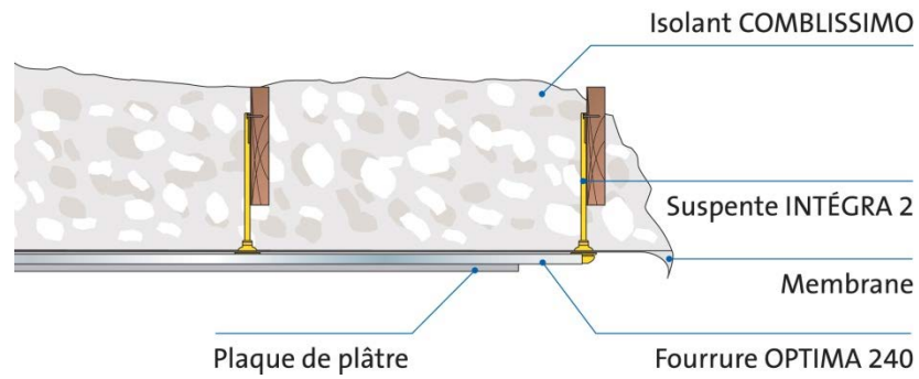
Figure 16 - Charpente en fermettes industrialisées pour comble perdu : Isolant en vrac soufflé mécaniquement - Mise en œuvre du procédé avec la suspenste Intégra2 (coupe en 2D)
