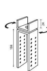
Support à tête pivotante
