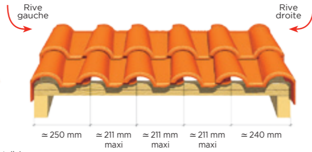
Pose avec rives à rabat
