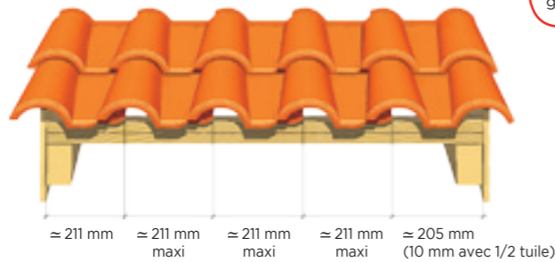
Pose avec rives individuelles verticales
