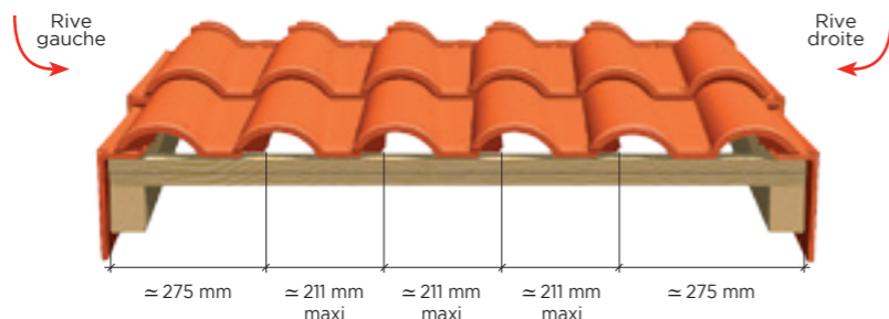
Pose avec rives individuelles verticales
